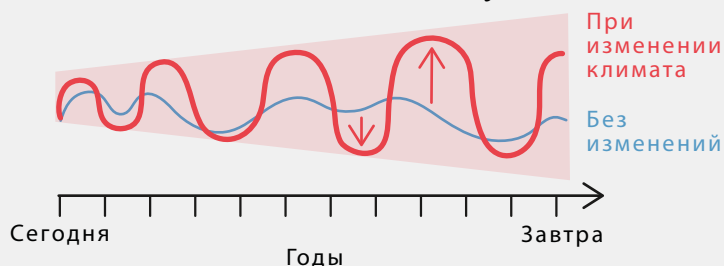
2 Более выраженные различия в водности от года к году
