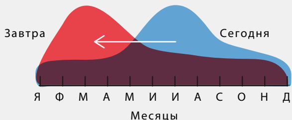
1 Изменение сезонного распределения стока
