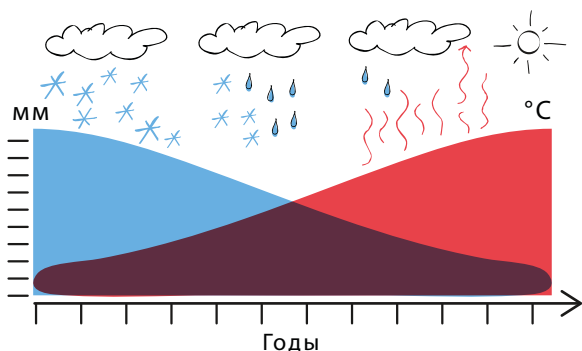
4 Сокращение устойчивого снежного покрова под влиянием потепления
